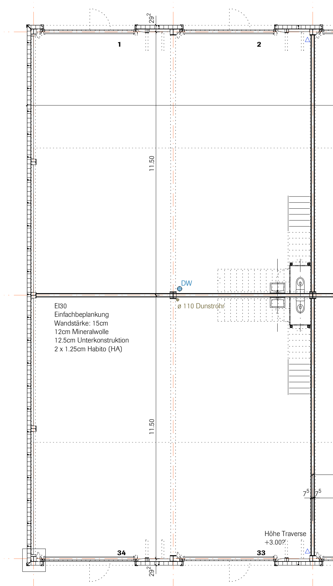
Grundriss EG
