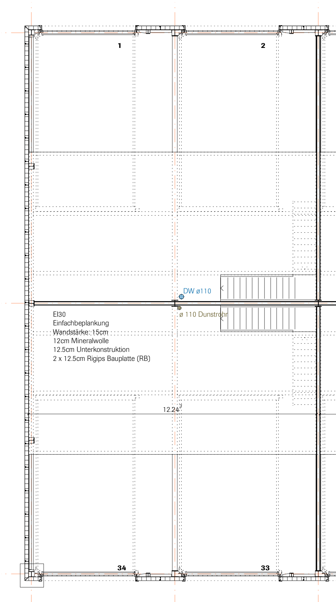
Grundriss OG
